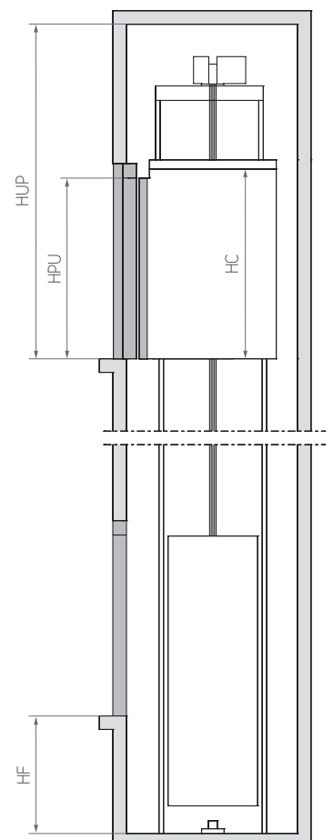
COUPE VERTICALE
